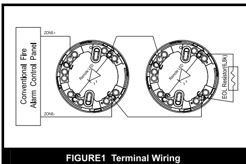
FIGURE1 Terminal Wiring
